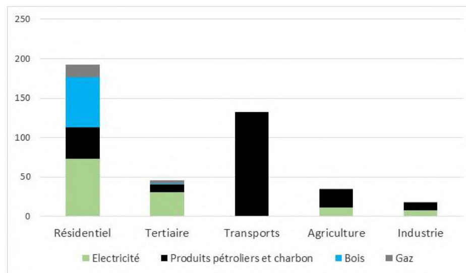
Figure 20 - Consommation par vecteur et par secteur (Prosper 2017)
