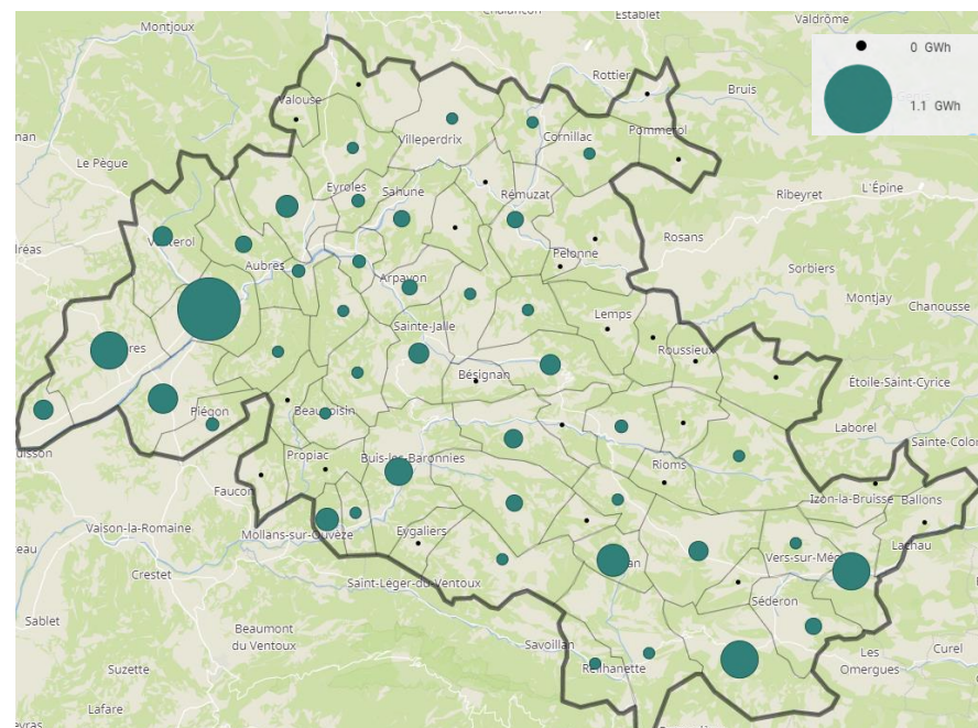
Figure 36 : Site de production de solaire photovoltaïque (Terristry)
