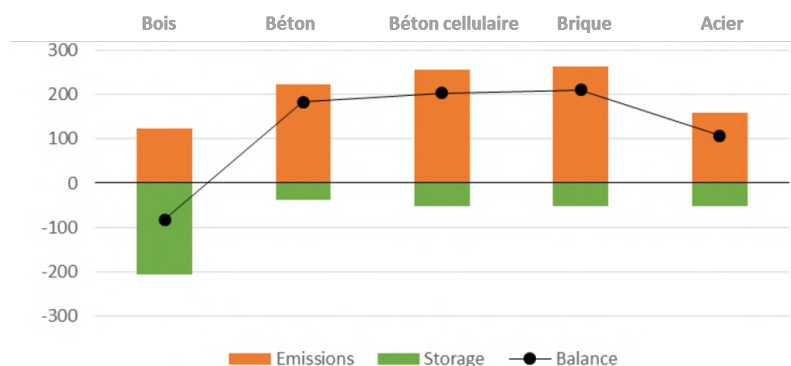
Figure 71 - Emissions et stockage carbone dans les matériaux de construction (CEI bois)
