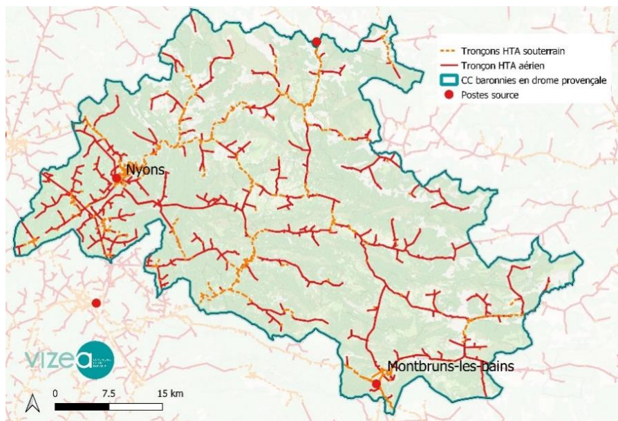
Figure 30 - Réseau de distribution d'électricité HTA (Vizea d'après les données d'ENEDIS, 2020)
