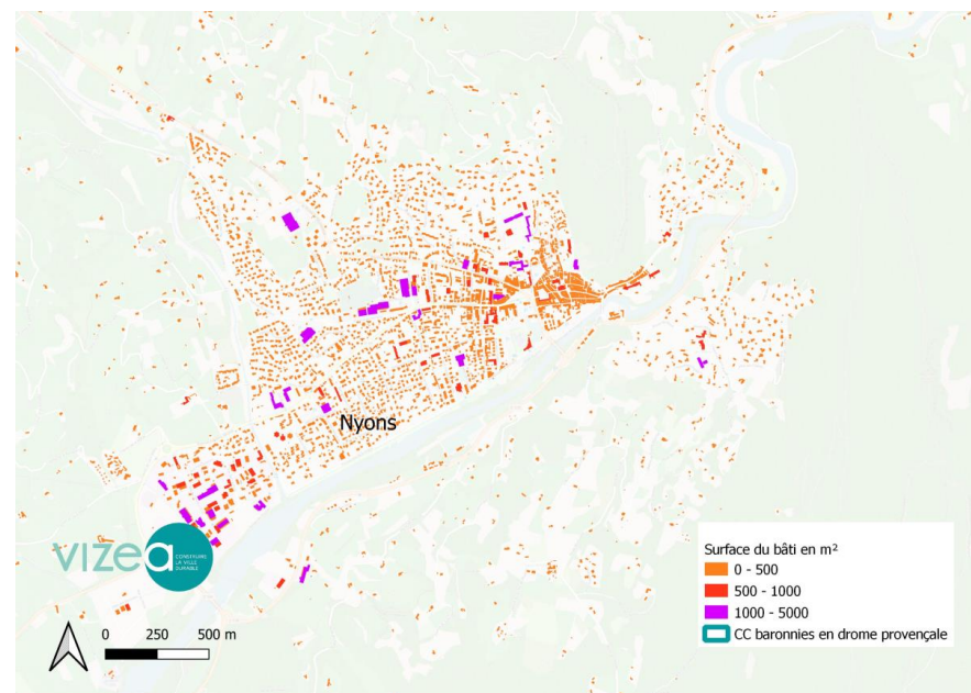
Figure 900 : Surface du bâti - Nyons
