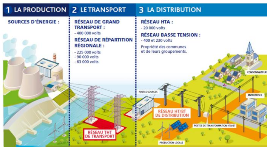
Figure 28 - Schéma explicatif sur le transport et la distribution d'énergie (sydela.fr)
