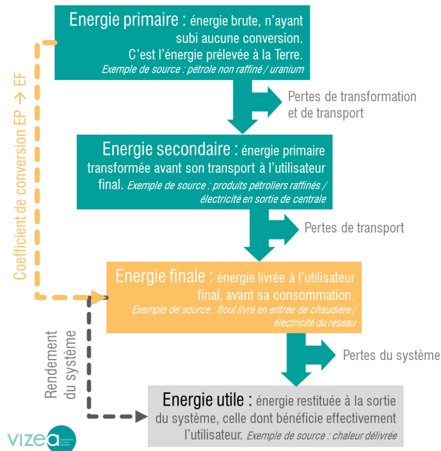
Figure 17 - Transformation de l'énergie (Vizea)
