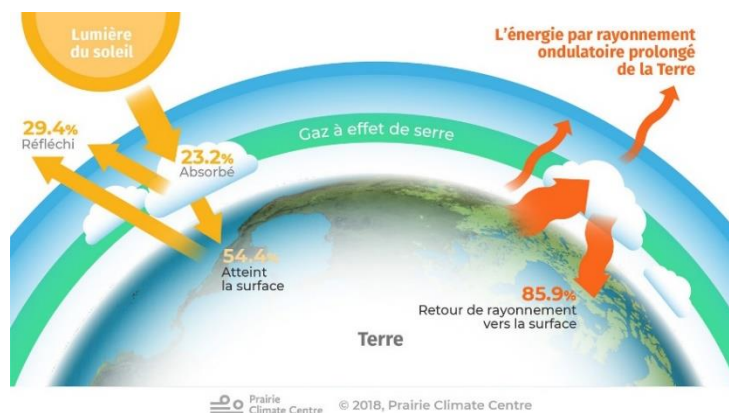
Figure 72 - Le phénomène de gaz à effet de Serre (Prairie Climate Centre, 2018)
