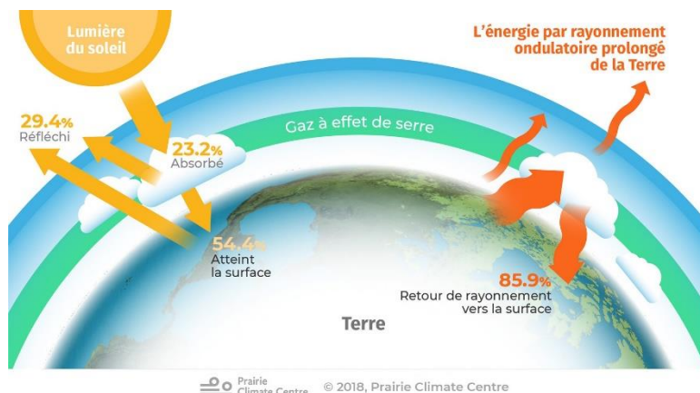
Figure 48 - Explication gaz à effet de Serre (Prairie Climate Centre, 2018)
