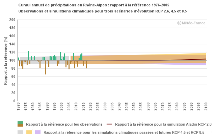
Figure 75 - Evolution des précipitations annuelles en Rhône-Alpes (Climat HD de Météo France)
