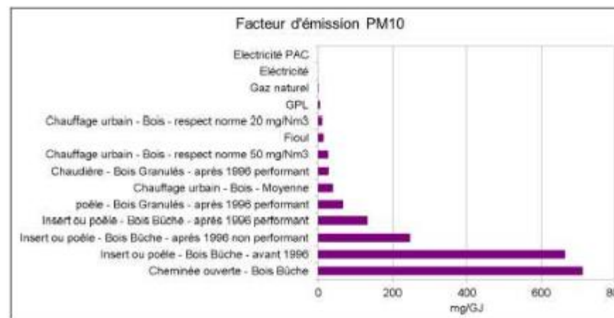
Figure 22 - Comparatif des facteurs d'émissions de PM 10 par la combustion (Source : SRCAE d'après ATMO Rhône-Alpes)
