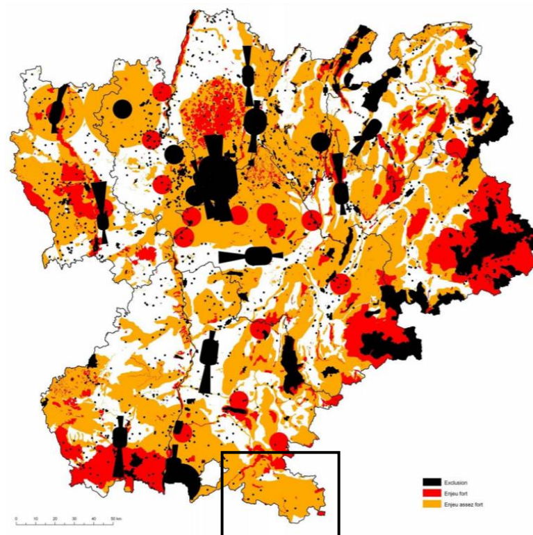
Figure 39 – Enjeu pour l'implantation d'éolienne sur le territoire (Schéma régional éolien Rhône-Alpes)
