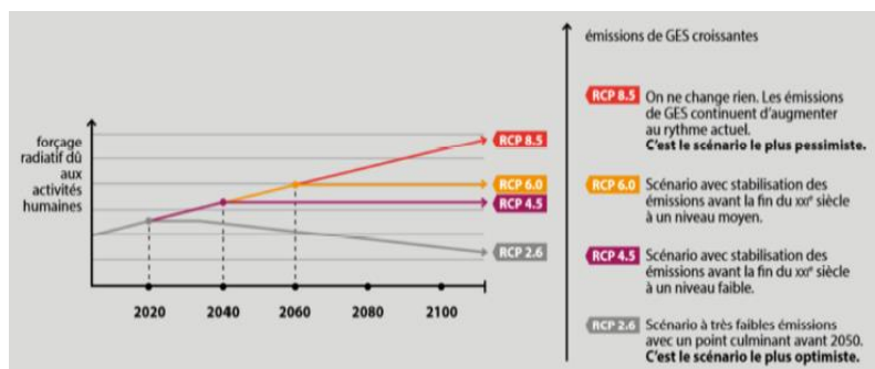
Figure 73 - Trajectoire des différents scénarios (RCP) – ONERC
