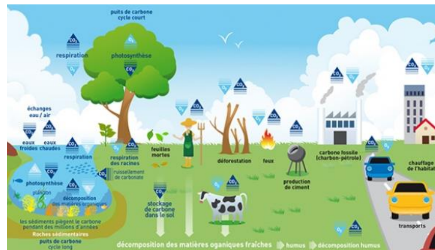
Figure 67 - Principe de séquestration naturelle du \text{CO}_2 (INRA)
