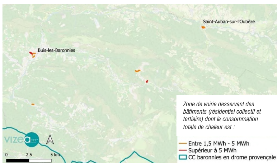
Figure 45 - Potentiel de développement des réseaux de chaleur – DREAL AURA
